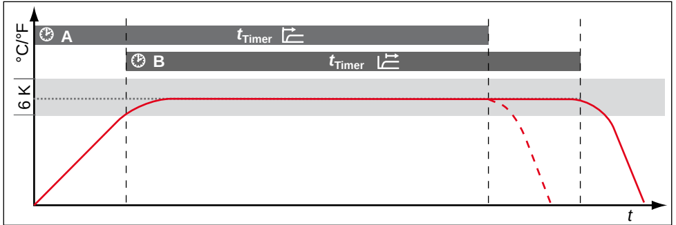
Fig. 27 Timer mode
